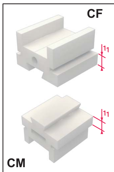
Cales de base «abs»
