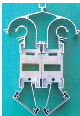
Profilé alu «haut de la structure»
