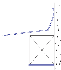
CALAGE POUR RAYONNEMENT EN PIGNON
