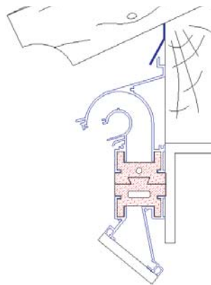
POSE EN SOUS FACE
